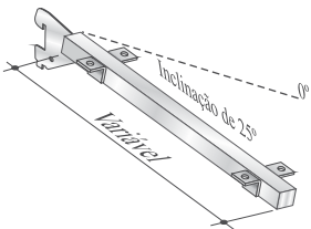
MCA-152 BRAÇO TUBO QUADRADO COM INCLINAÇÃO P/ PRATELEIRA DE MADEIRA C/ CANTONEIRAS
