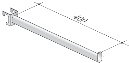
MCA-181 BRAÇO PARA EXPOSIÇÃO FRONTAL COM ENCAIXE PARA PONTALETE
