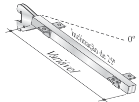
MCA-154 BRAÇO TUBO QUADRADO PARA PRATELEIRA DE MADEIRA COM CANTONEIRAS INCLINADO
