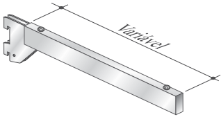
MCA-195 BRAÇO TUBO RETANGULAR PARA PRATELEIRA DE VIDRO COM VENTOSAS
