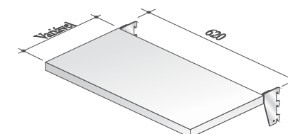
MCA-205 PRATELEIRA DE CHAPA METÁLICA - COM BRAÇO FACA 3 DENTES
