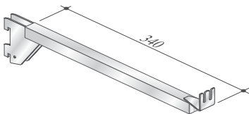
MCA-156 BRAÇO SUPORTE COM MÃOZINHA
