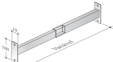
MCA-170 TRAVESSA DE FIXAÇÃO COM REGULAGEM
