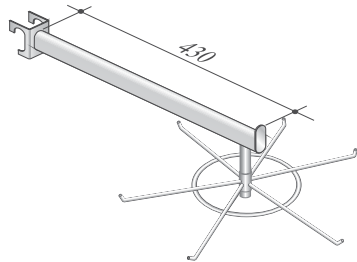
MCA-182 BRAÇO GIRATÓRIO PARA CINTOS E GRAVATAS COM ENCAIXE PARA PONTALETE
