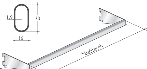
MCA-173 PONTALETE COM APOIO FIXO
