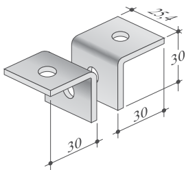
MCA-163 CANTONEIRA PARA BRAÇOS
