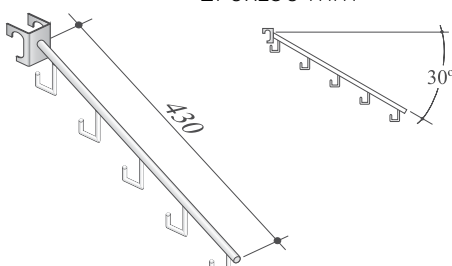
MCA-180 BRAÇO INCLINADO COM GANCHO
