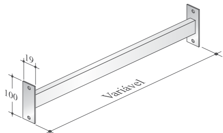
MCA-167 TRAVESSA DE FIXAÇÃO
