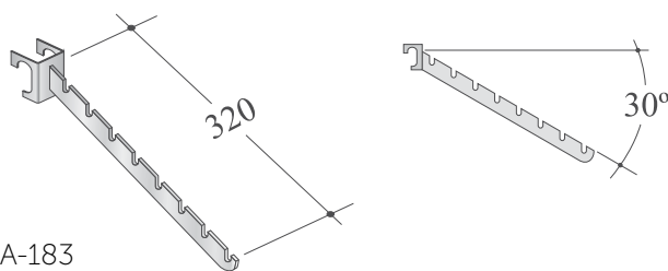
MCA-183 BRAÇO INCLINADO TIPO SERRA PARA PONTALETE
