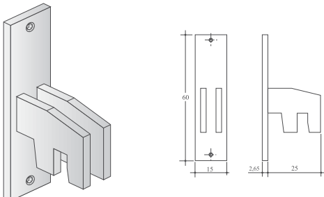
MCA-161 FIXADOR FRONTAL PARA DIVISÓRIAS
