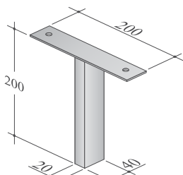
MCA-164 CONEXÃO DE TETO
