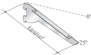
MCA-155 BRAÇO FACA INCLINÁVEL PARA PRATELEIRA DE MADEIRA COM CANTONEIRAS
