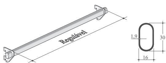
MCA-172 PONTALETE REGULÁVEL
