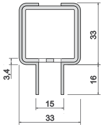
MCC-160 COLUNA 30 X 30 C/ CAPA ESTAMPADA 1 LADO
