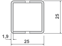
MCC-163 COLUNA 25 X 25 S/ CAPA ESTAMPADA 2 LADOS
