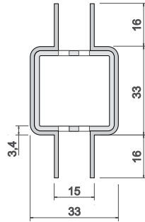
MCC-162 COLUNA 30 X 30 C/ CAPA ESTAMPADA 2 LADOS
