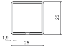
MCC-165 COLUNA 25 X 25 S/ CAPA ESTAMPADA 1 LADO
