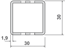
MCC-159 COLUNA 30 X 30 S/ CAPA ESTAMPADA 2 LADOS
