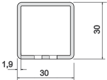
MCC-161 COLUNA 30 X 30 S/ CAPA ESTAMPADA 1 LADO
