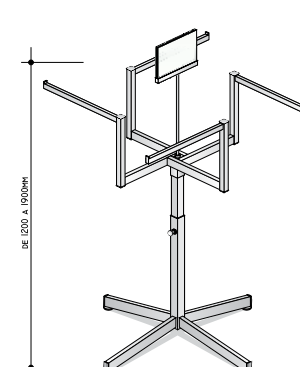
MCE-159 ARARA CRUZ COM REGULAGEM
