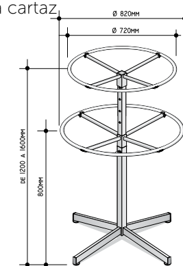
MCE-153 ARARA CRUZ CIRCULAR COM REGULAGEM DE ALTURA
