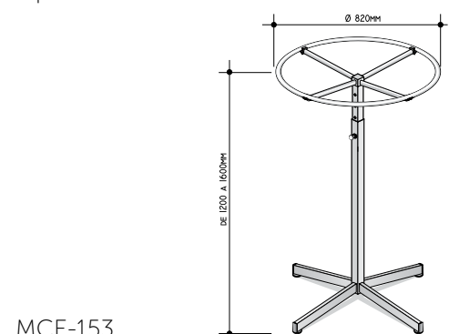
MCE-153 ARARA CRUZ CIRCULAR COM REGULAGEM DE ALTURA
