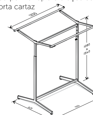
MCE-160 ARARA PARALELA COM REGULAGEM DE ALTURA
