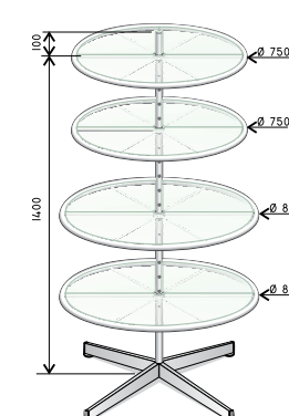
MCE-174 ARARA REDONDA CALÇADPS 4 ANDARES - VIDRO OPCIONAL
